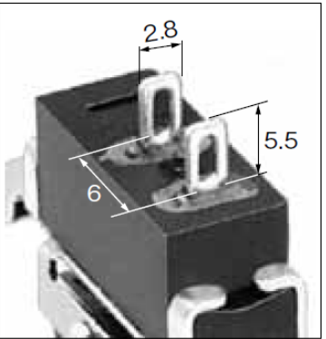
半田端子
