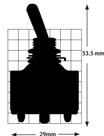
シルエット (AWTA21)
