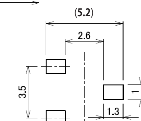
取付ランド寸法 (S=5/1) (共通)
