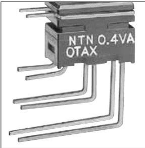
PWB バーティカル端子 (2 極 ON-ON)
