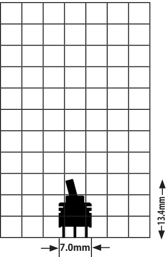
シルエット (NTD12)
