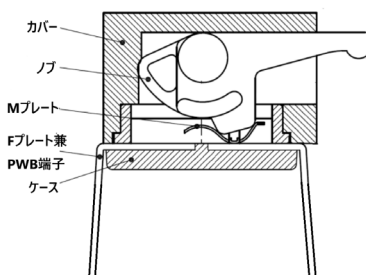
スルーホール実装形
