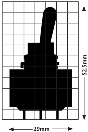
シルエット (BTD01)
