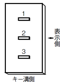
■ 端子番号図
