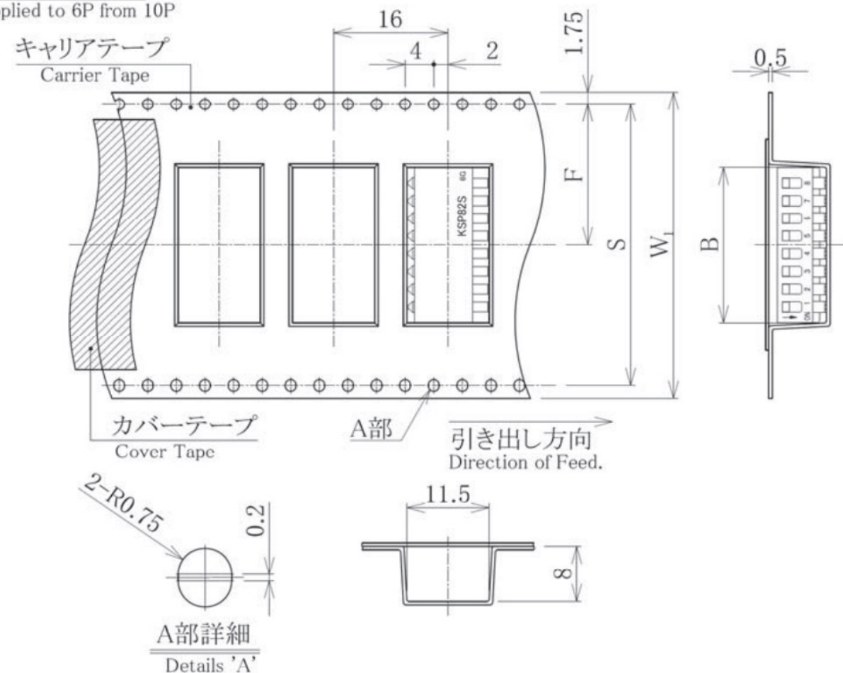
各部の寸法 (mm)
