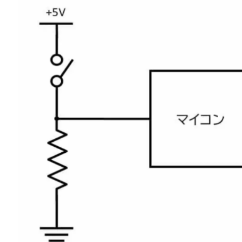
プルダウン回路
