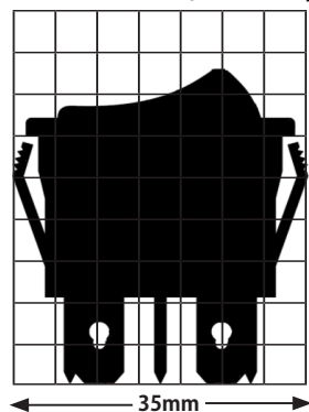
シルエット (TLD15C1)
