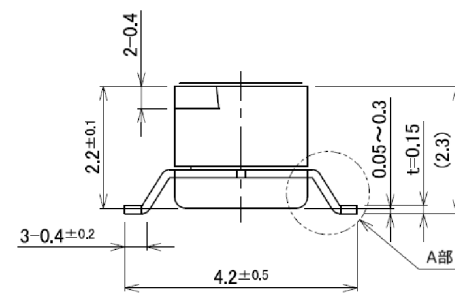
側面（共通）
