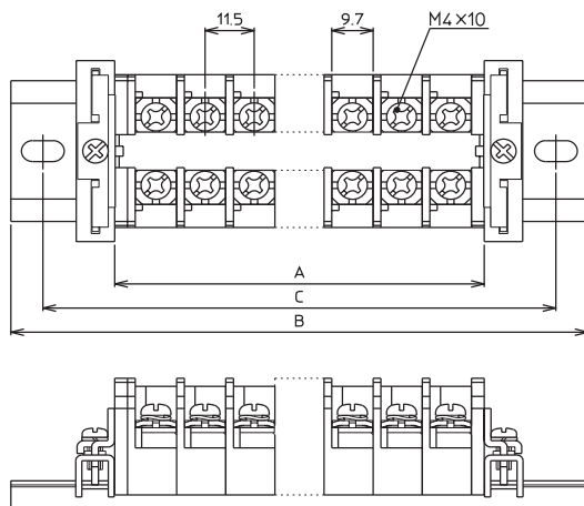
外観図 (単位: mm)
